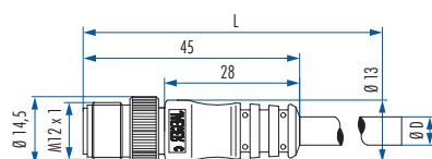
Kupplungssteckverbinder
