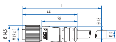
Kabelsteckverbinder
