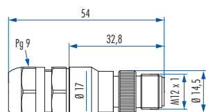
Kupplungssteckverbinder (4 – 8 mm)
