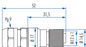
Kabelsteckverbinder (4 – 8 mm)
