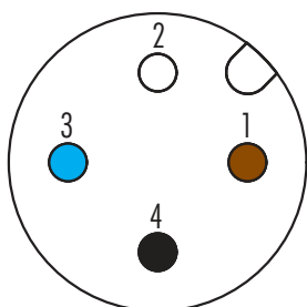
4 Kontakte
