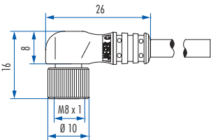
Winkelsteckverbinder (Buchse)
