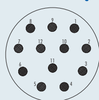
Kontaktnumerierung
