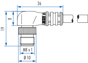
Winkelsteckverbinder (Stift)
