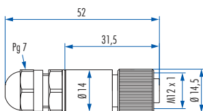
Kabelsteckverbinder (3 – 6,5 mm)
