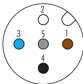
5 Kontakte
