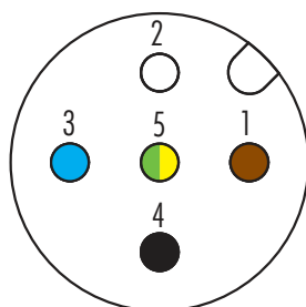
5 Kontakte
