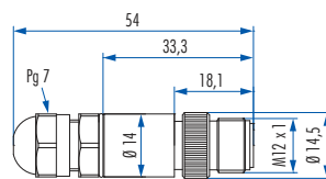
Kupplungssteckverbinder (3 – 6,5 mm)
